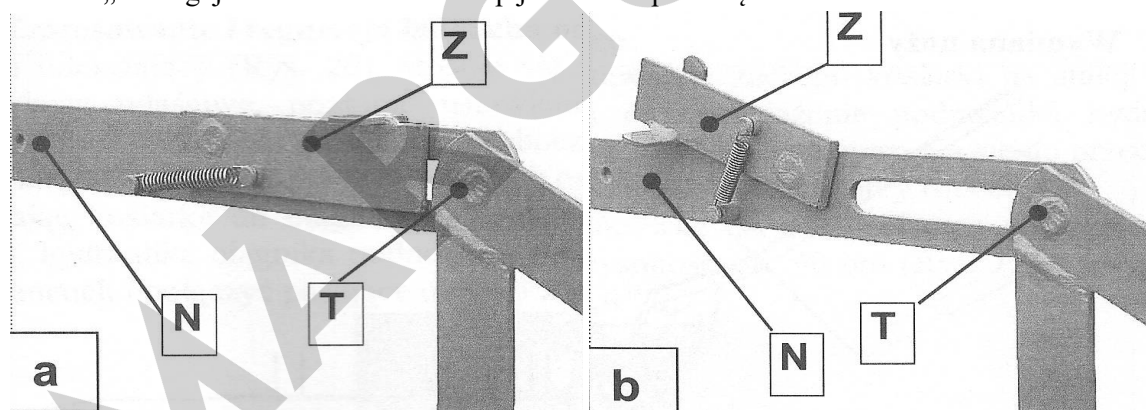
Pav. 9. Spragtuko „Z“ pervedimas į padėtį: a) transportavimo; b) darbinę.
