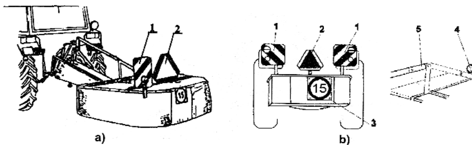
Pav. 8. Šienapjovė transportavimo padėtyje su išpėjamaisiais ženklais.
