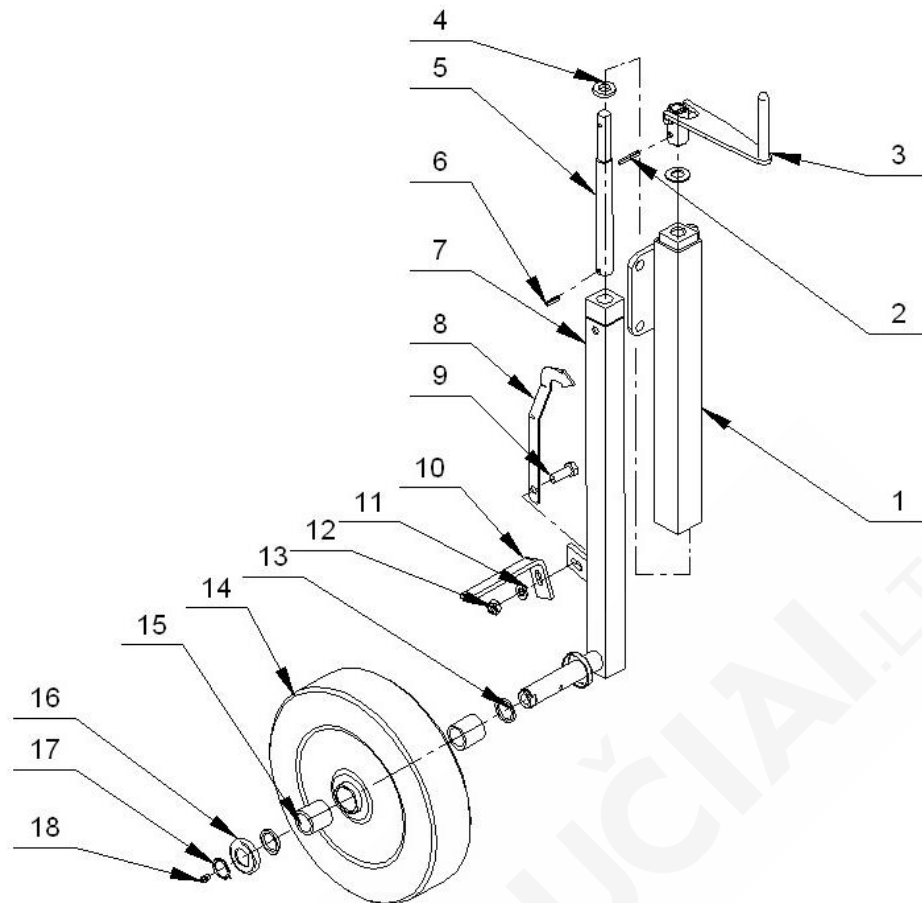
Rys.10 Zespół koła podporowego GT-15. (Tabela 10)
