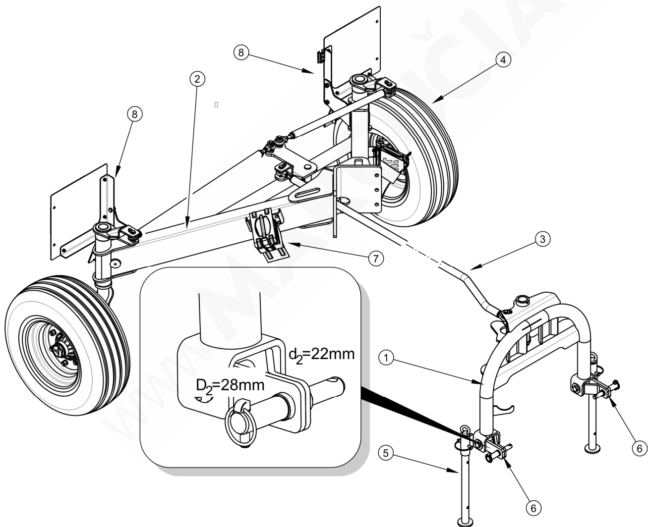
RYСУNEK 3.2 Budowa układów jezdny i zaczepowy
