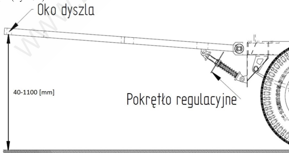
Rys. 6.2 Sposób regulacji wysokości oka dyszla
