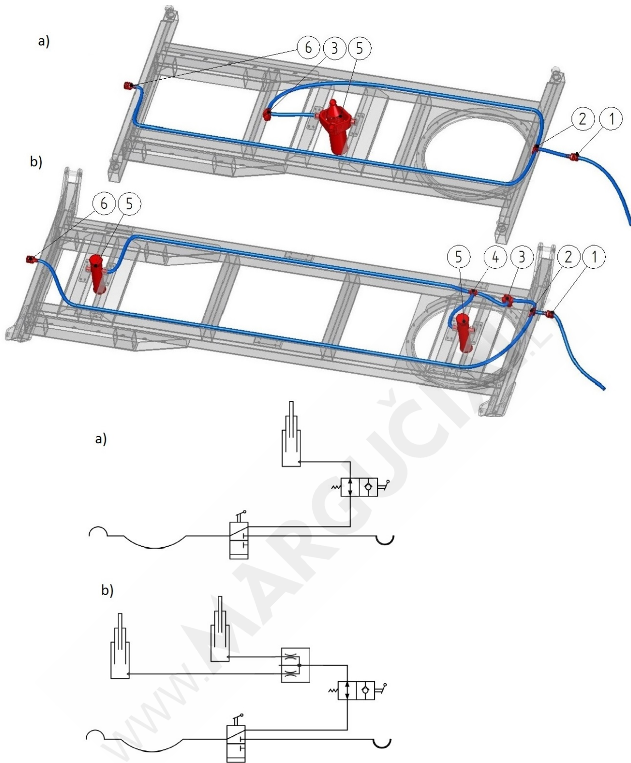
Rys. 4.3 Budowa i schemat hydraulicznej instalacji: a) trójstronnego wywrotu, b) dwustronnego wywrotu 1- wtyka szybkozłączna; 2- zawór trójdrogowy; 3- zawór odcinający; 4- dzielnik strumienia; 5- siłownik teleskopowy; 6- gniazdo szybkozłączna
