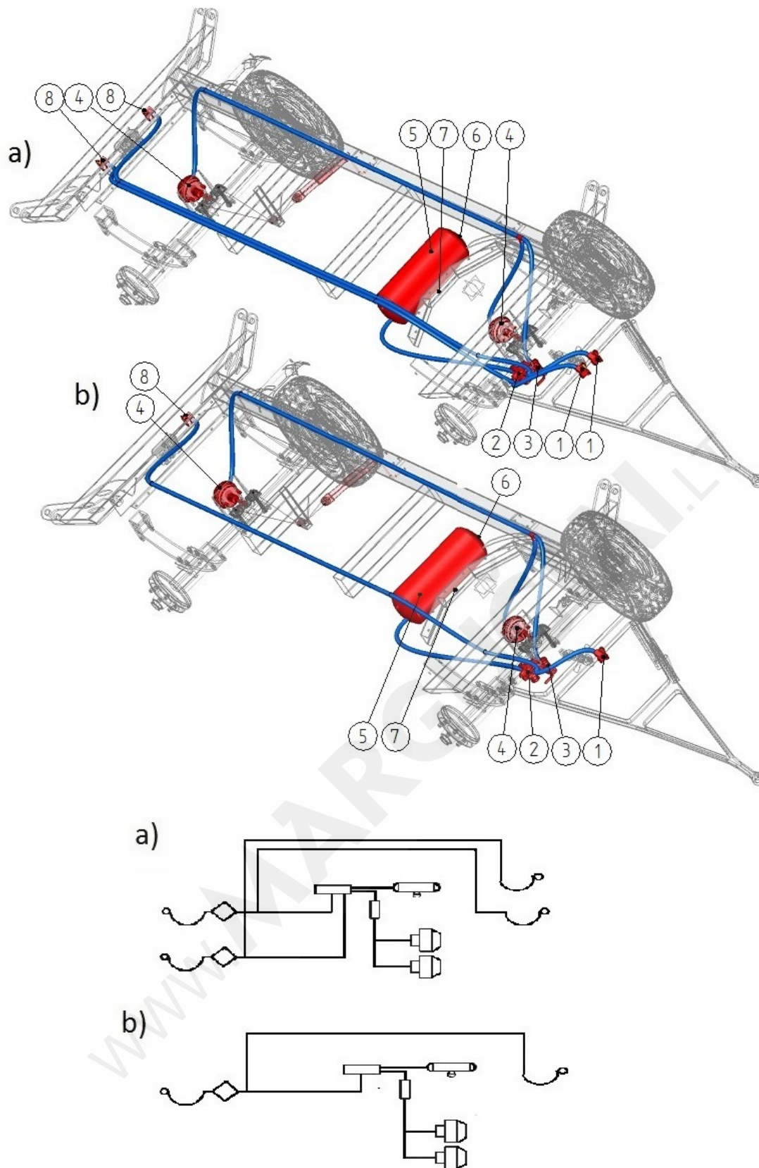
Rys.4.4 Budowa i schemat pneumatycznej instalacji hamulcowej: a) dwuprzewodowej, b) jednoprzewodowej 1- złącze pneumatyczne z wbudowanym (lub oddzielnym) filtrem powietrza; 2- zawór sterujący; 3- regulator siły hamowania; 4- siłownik pneumatyczny; 5- zbiornik powietrza; 6- złącze kontrolne zbiornika powietrza; 7- zawór odwadniający; 8- złącze pneumatyczne drugiej przyczepy
