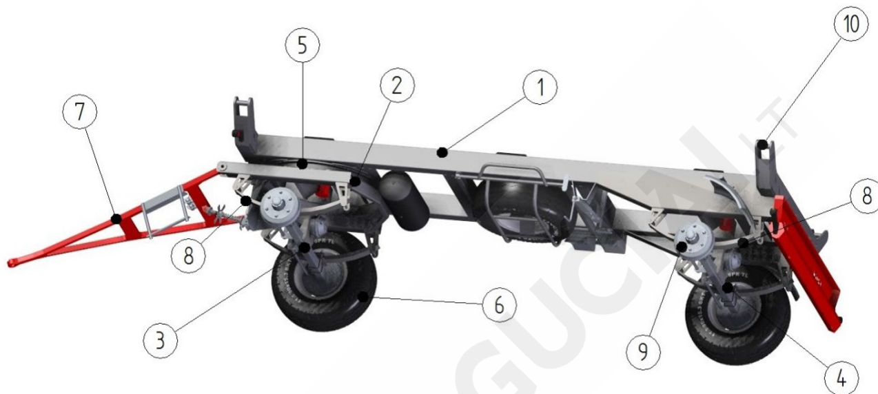
Rys. 4.1 Podwozie przyczepy PD. 1- rama główna; 2- rama wózka obrotnicy; 3- przednia oś jezdna; 4- tylna oś jezdna; 5- wieńiec obrotu (obrotnica); 6- koło jezdne; 7- dyszel; 8- resor piórowy; 9- piasto-bęben; 10- sworzień/kula wywrotu.
