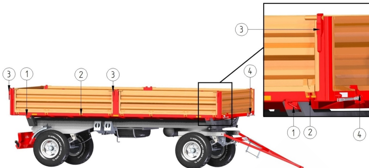
Rys. 5.3 Zamki i sworznie wywrotu skrzyni ładunkowej. 1- sworznię wywrotu; 2- zamek dolny; 3- zamek górny; 4- centralny rygiel zamków dolnych
