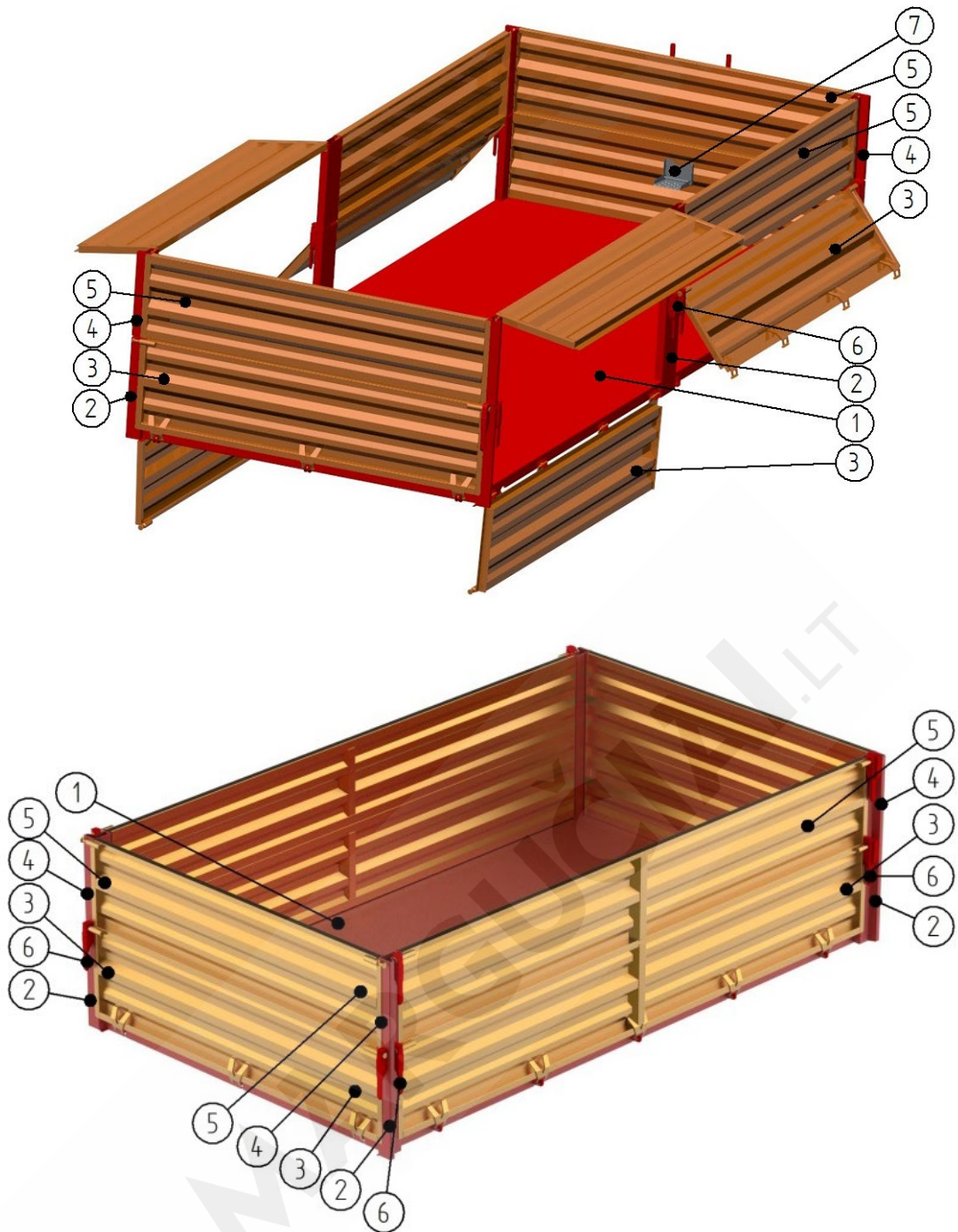
Rys. 4.2 Skrzynia ładunkowa przyczepy PD. 1- podłoga; 2- słupki ścian; 3- ściany; 4- słupki nadstaw; 5- nadstawy; 6- zamki ścian; 7- stopień naburtowy.
