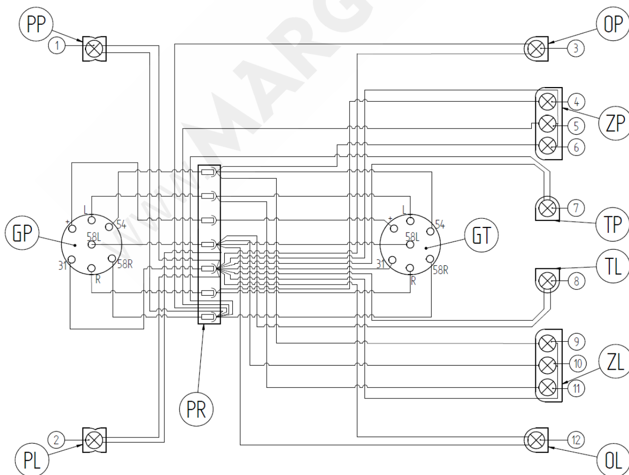
Rys. 4.8 Schemat instalacji elektrycznej (oświetleniowej).
