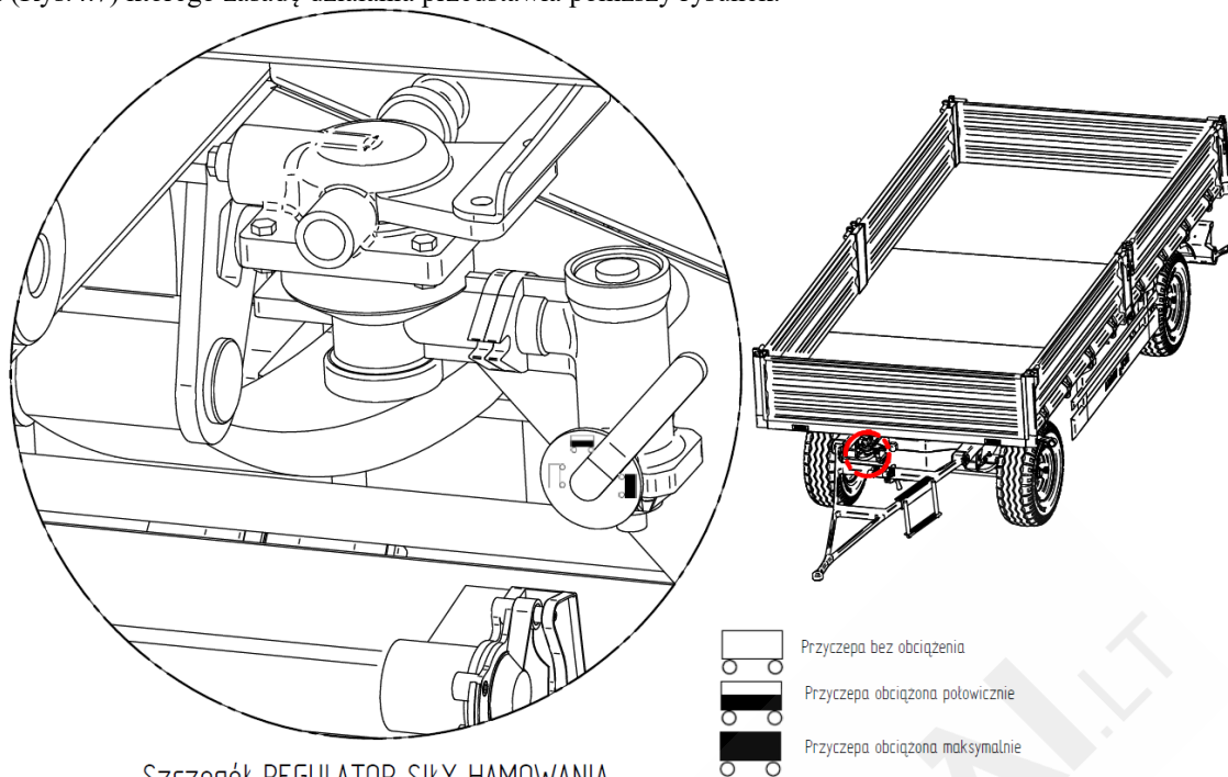
Rys. 4.7 Ręczny regulator siły hamowania.
