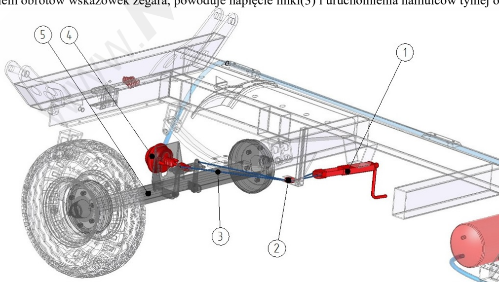
Rys. 4.6 Budowa hamulca postojowego.
