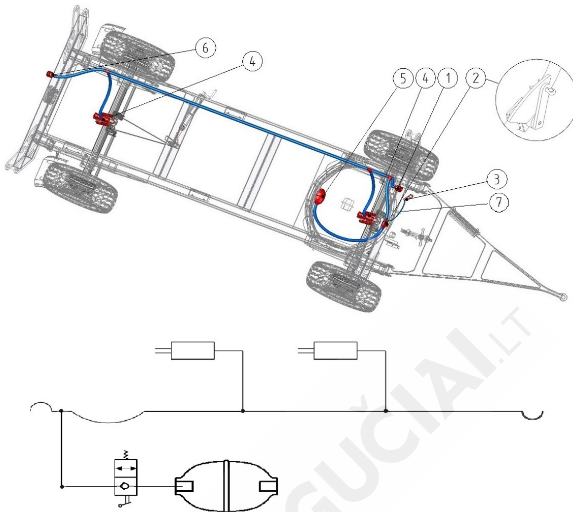
Rys.4.5 Budowa i schemat hydraulicznej instalacji hamulcowej.
